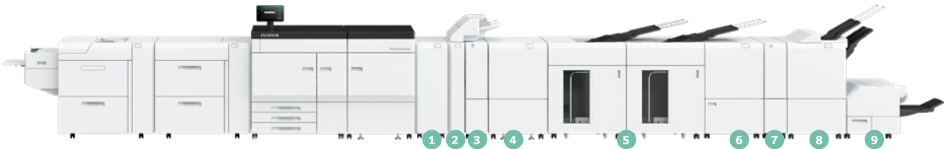
Configuração completa: L 10462 x P 1104 x A 1786 mm
